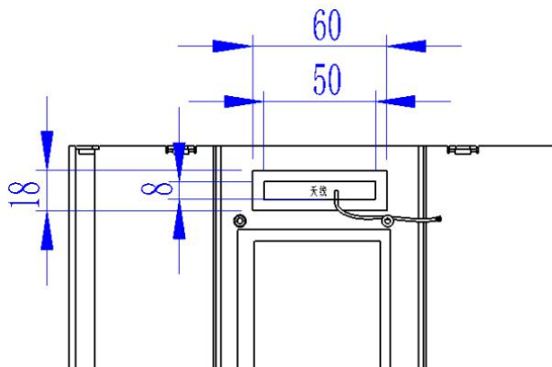
图 4 Antenna position
