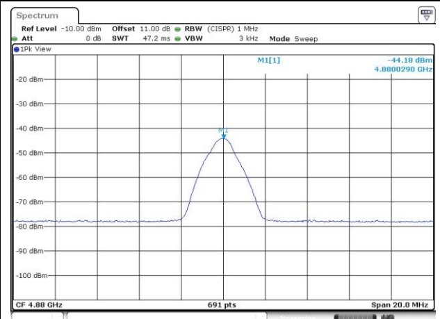
4880MHz - AV
