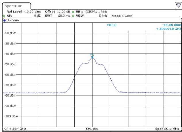
4804MHz - AV
