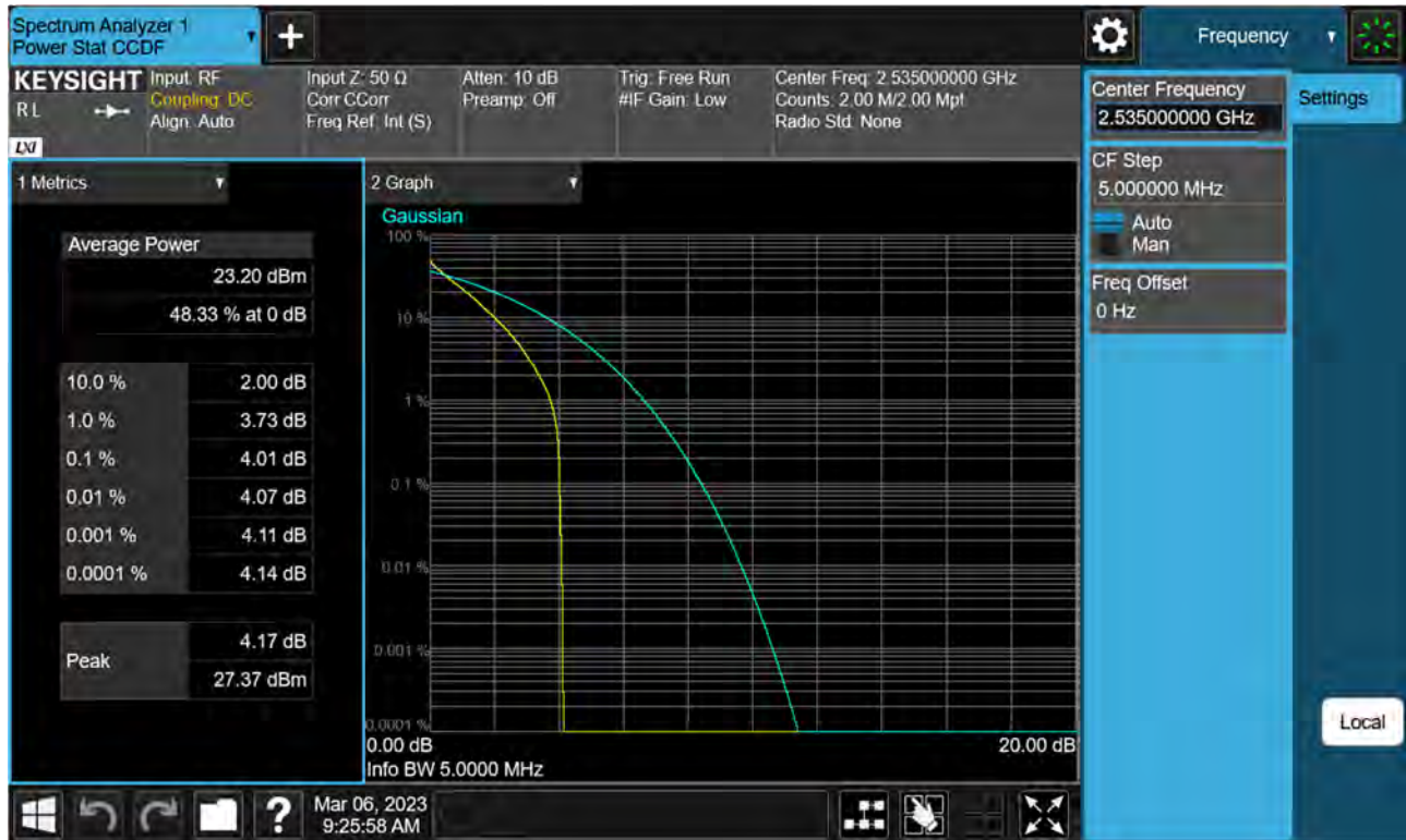
Sub6 n7. PAR Plot (5 M BW_Ch.507000_ BPSK)
