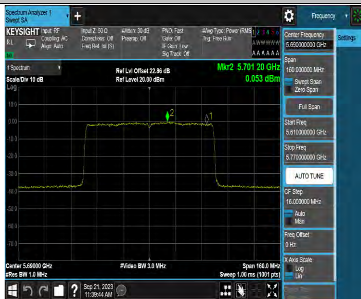
11AX80MIMO_Ant3_5690_UNII-2C
