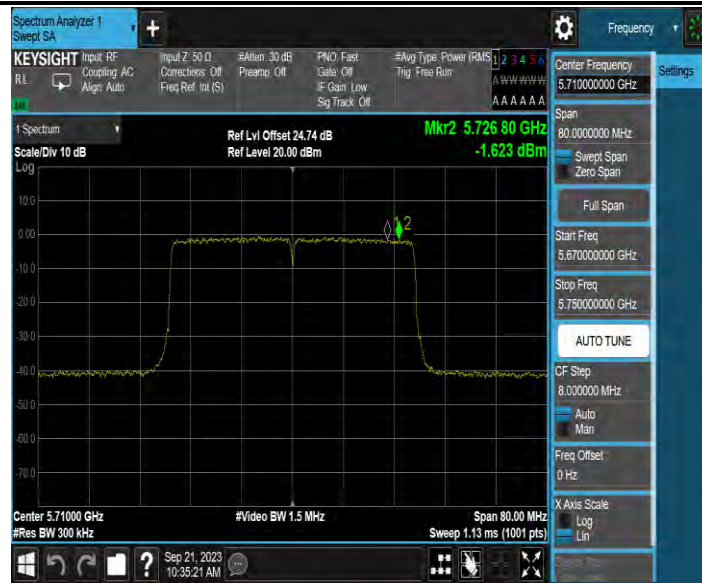
11AX40MIMO_Ant2_5710_UNII-3
