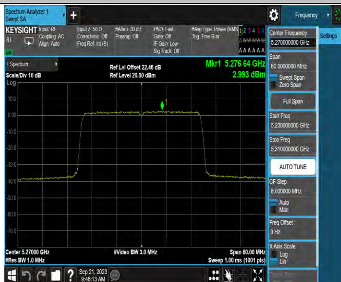
11AX40MIMO_Ant3_5270
