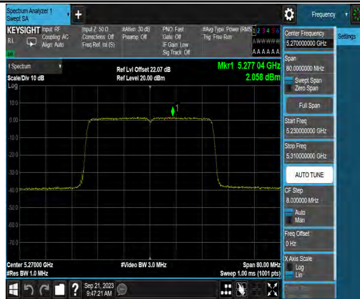
11AX40MIMO_Ant4_5270
