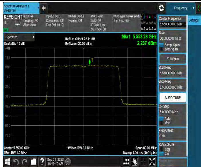
11AX40MIMO_Ant4_5550
