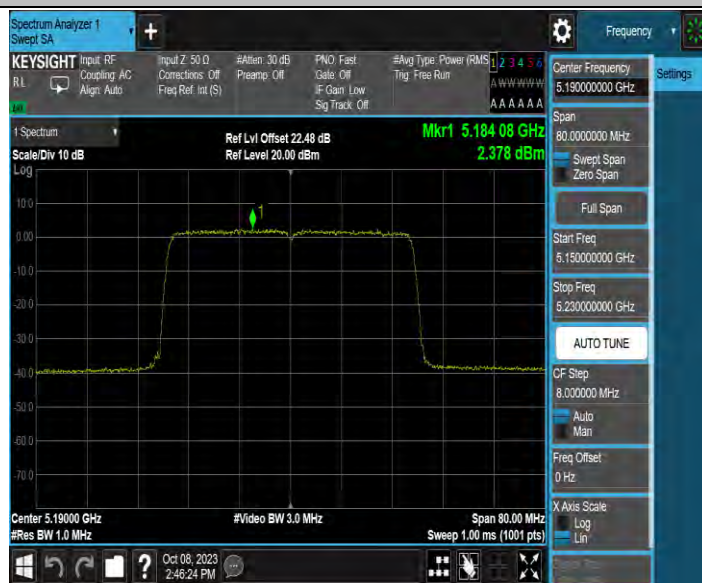
11AX40MIMO_Ant3_5190
