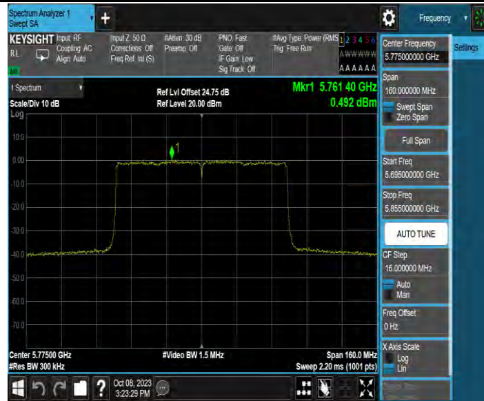
11AX80MIMO_Ant4_5775
