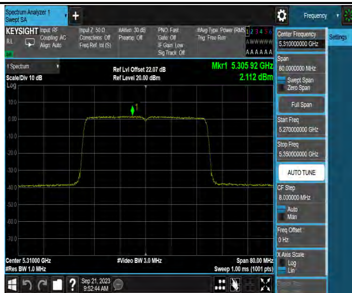
11AX40MIMO_Ant4_5310
