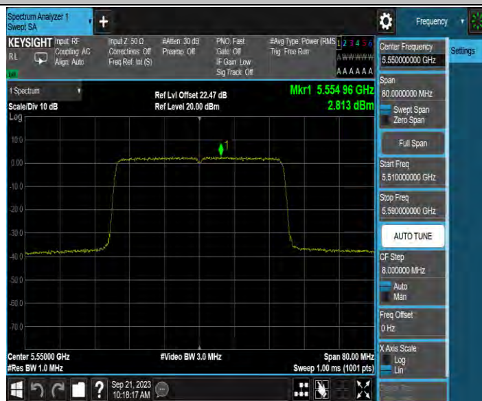
11AX40MIMO_Ant3_5550
