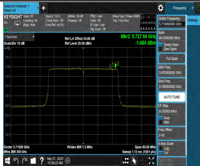
11AX40MIMO_Ant4_5710_UNII-3
