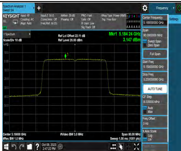
11AX40MIMO_Ant4_5190
