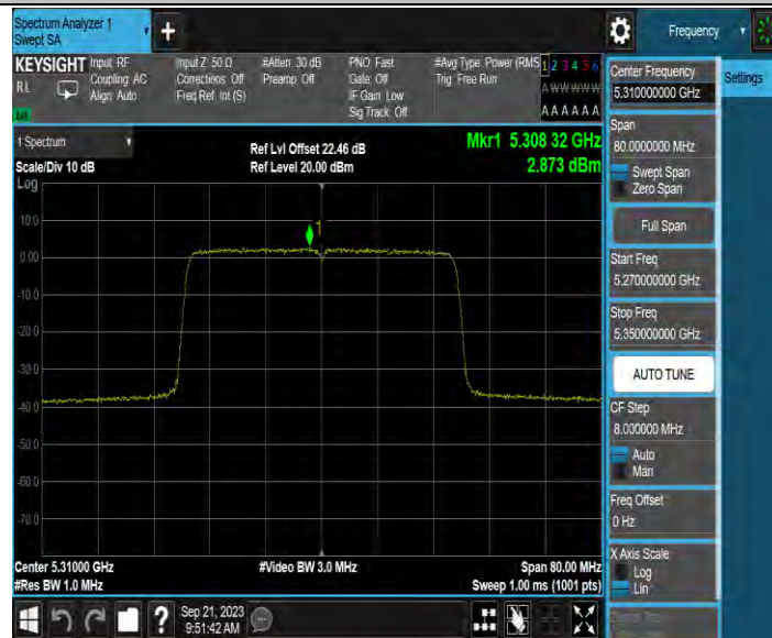
11AX40MIMO_Ant3_5310
