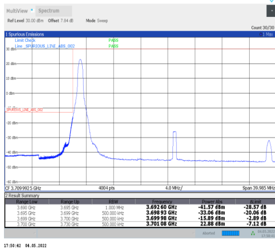
1-N78-3700-3800--30-30-L-4-CP-QPSK-Edge_1RB_L eft-1@0-Ant0-PASS-see graph
