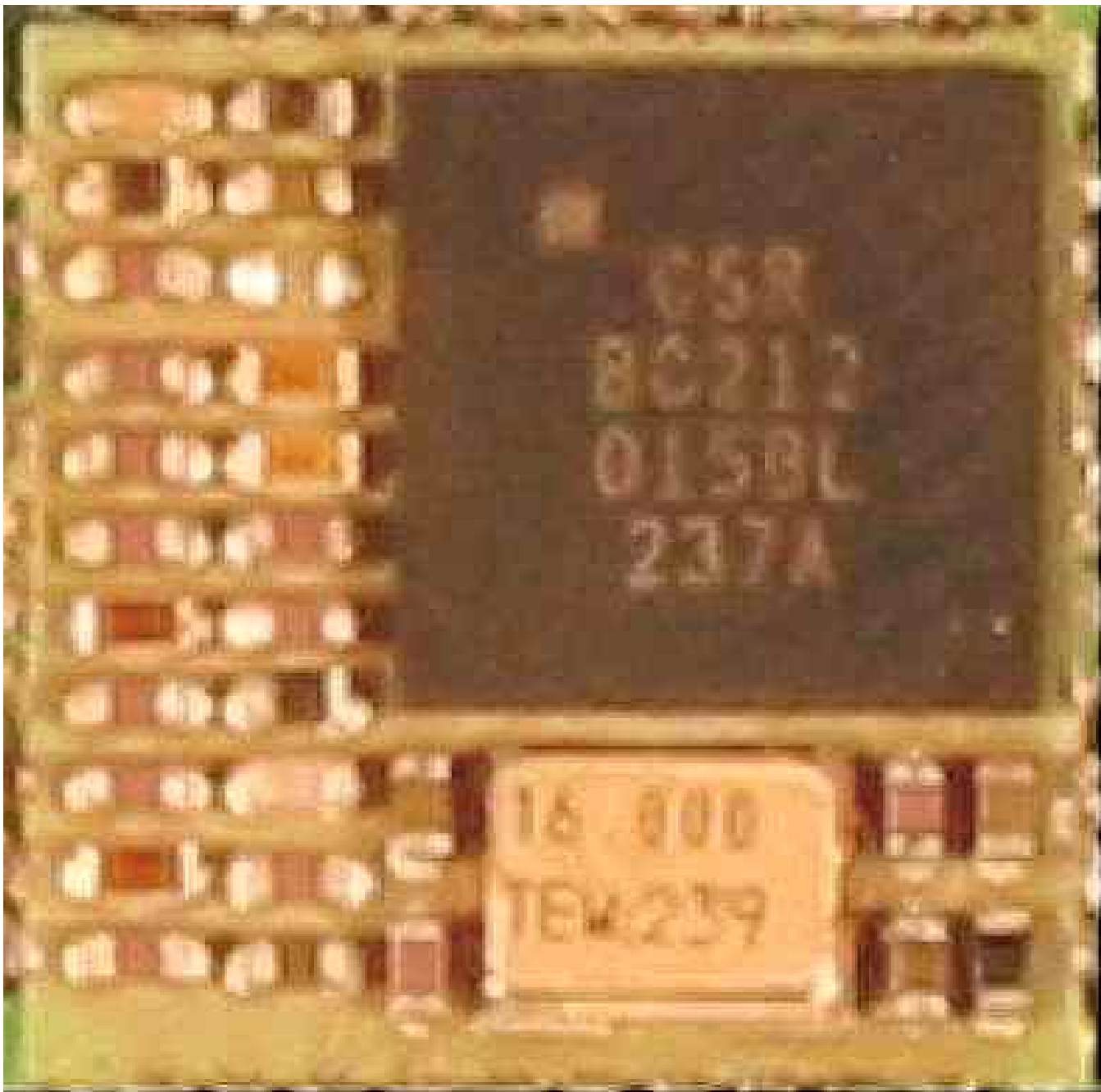
Radio Module (Internal)
